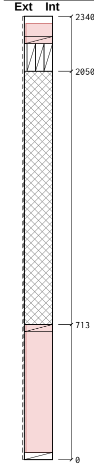
Section A-A
